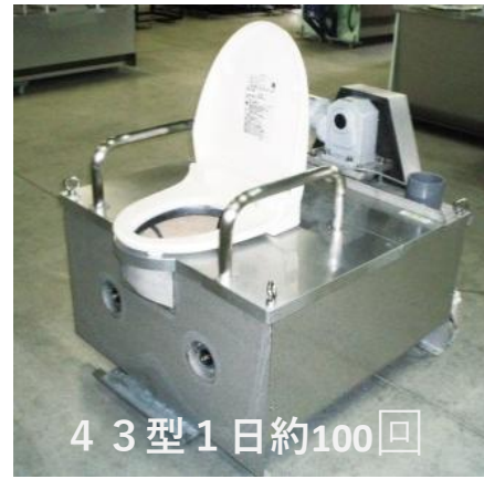
本体 SW型
